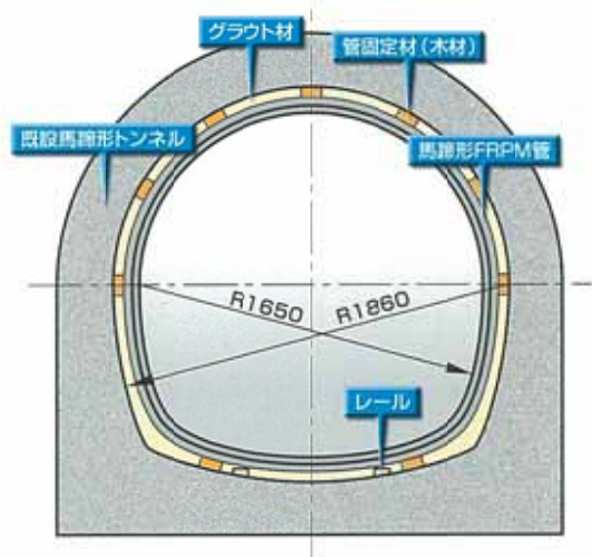
既設トンネル:2r-1860馬蹄形トンネル 内挿管:2r-1650馬蹄形FRPM管 掘工延長:510.27m
